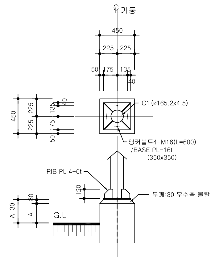
1/S 기둥 상세도 축척: 1/30
