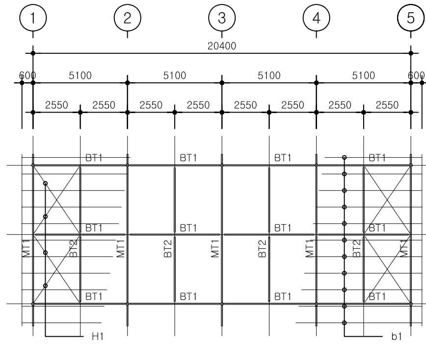
2 지붕 구조평면도 축척: 1/200
