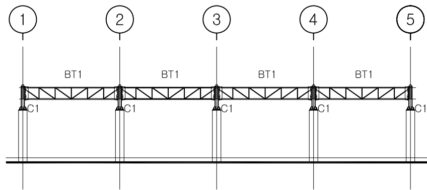
4 'B'열 구도 입면도 축척: 1/200
