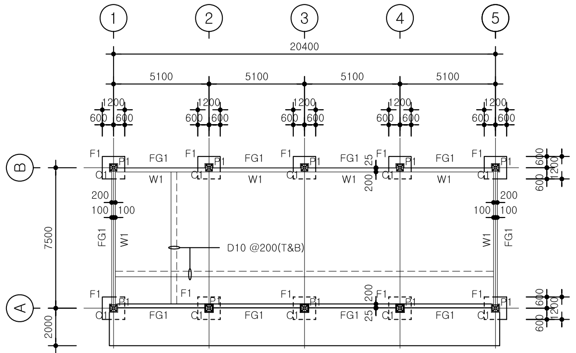
1 기초 바닥 구조평면도 축척: 1/200
