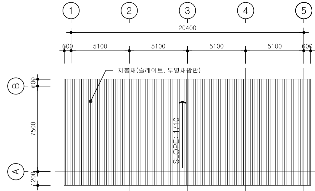
2 지붕 평면도 축척: 1/200
