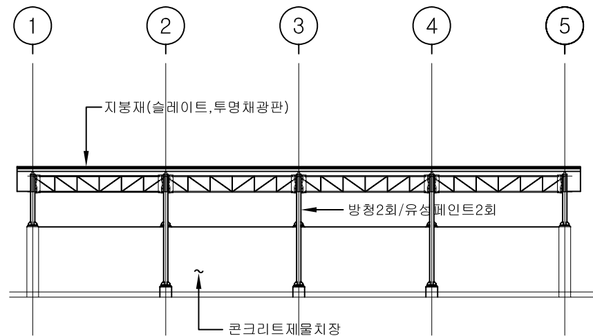
3 정면도 축척: 1/200
