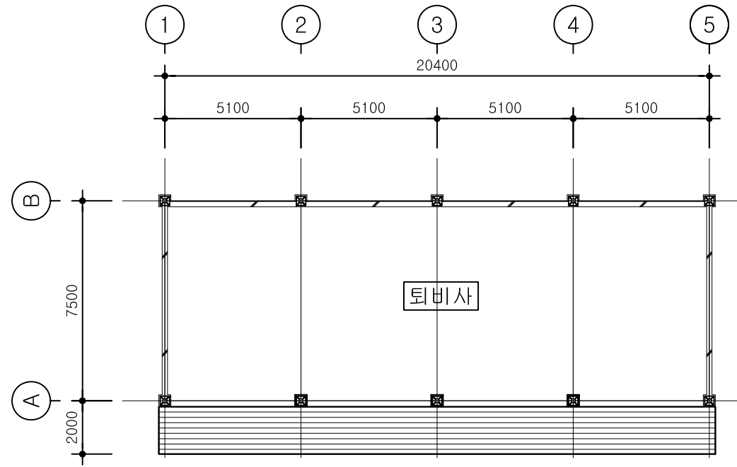
1 평면도 축척: 1/200
