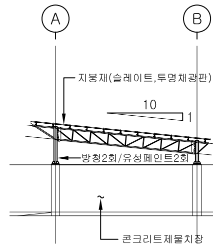
4 우측면도 축척: 1/200
