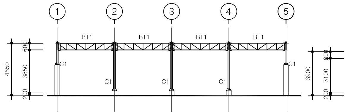
3 'A'열 구도 입면도 축척: 1/200
