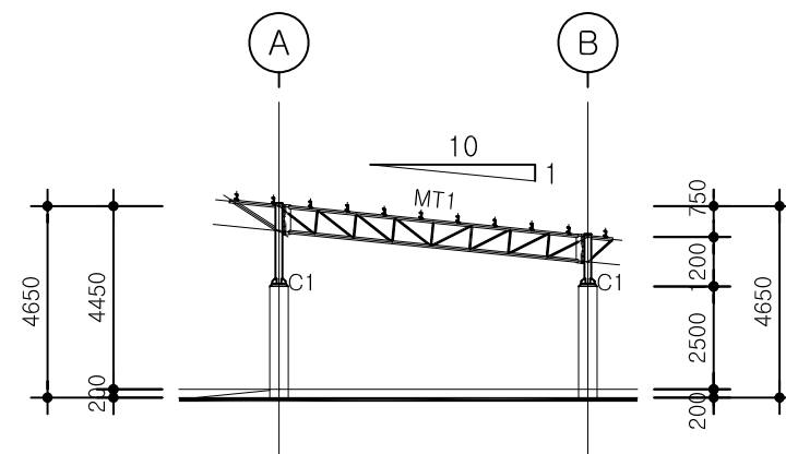
5 '1-5'열 구도 입면도 축척: 1/200
