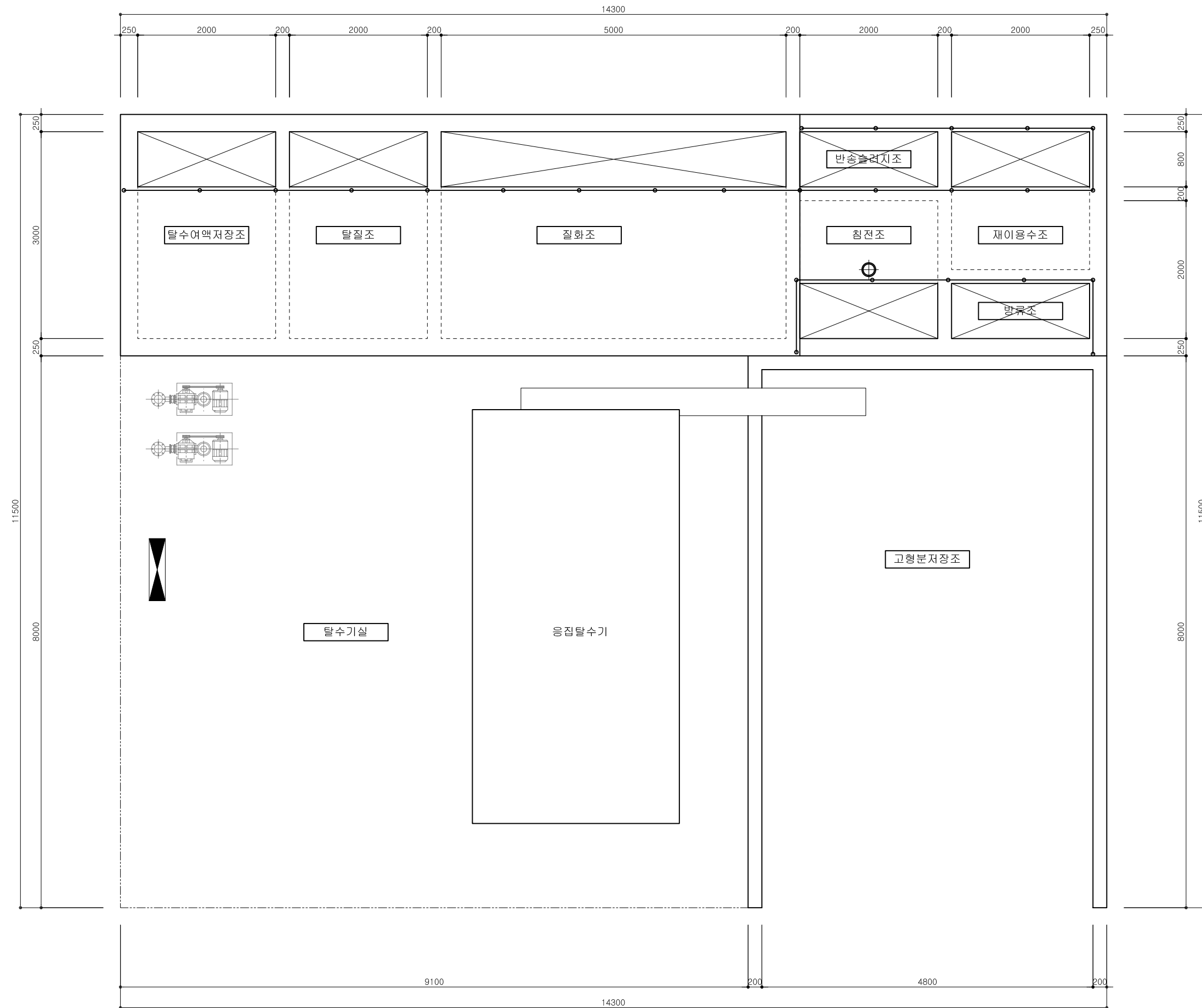
1 정화처리시설 평면도 축척: 1/60
