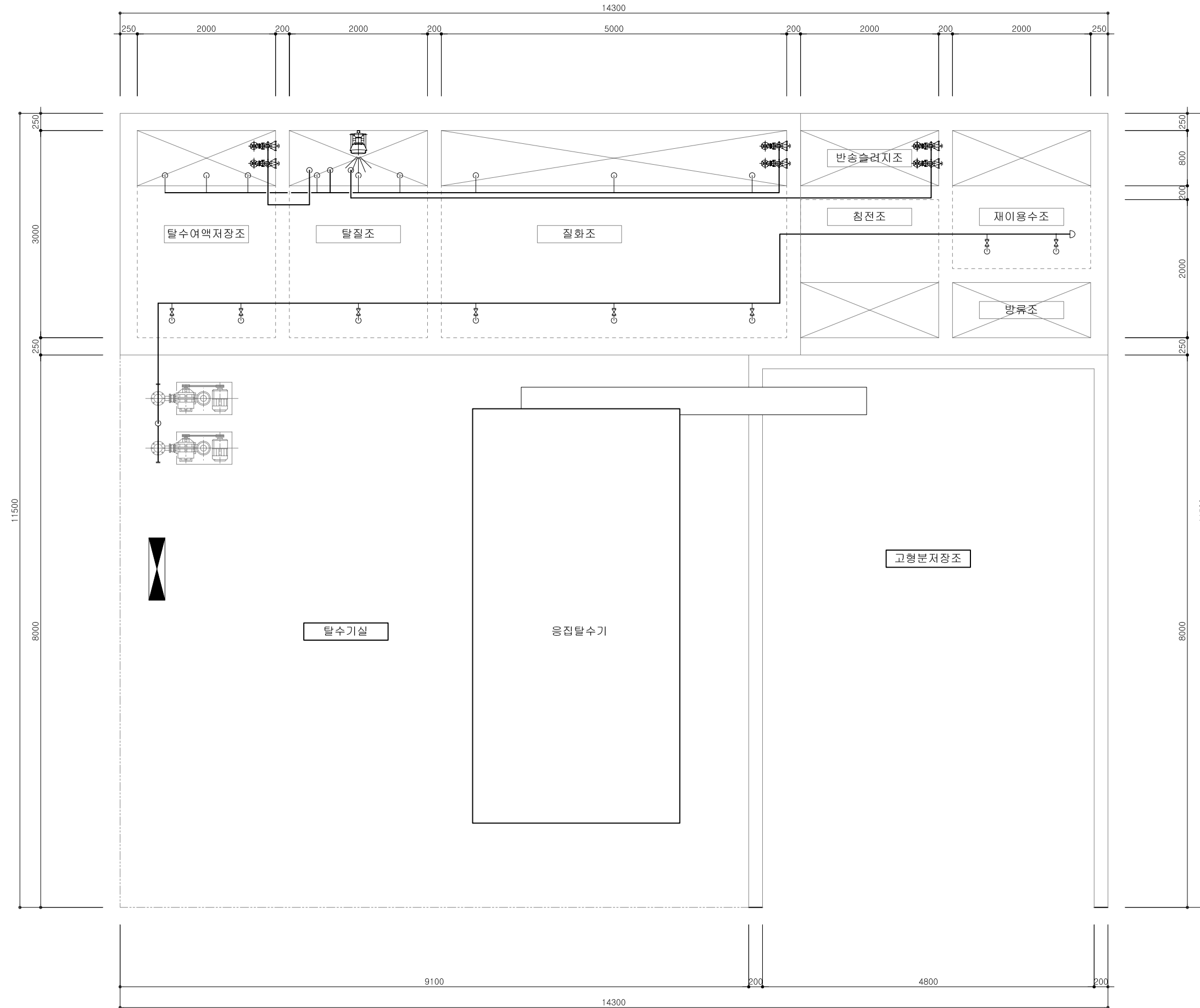
1 상부 배관 평면도 축척: 1/60
